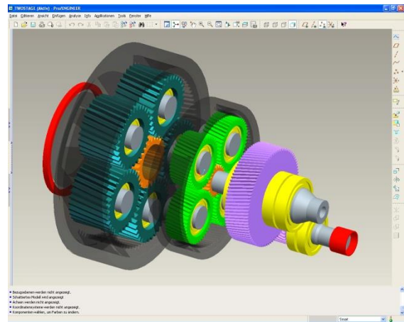
Bild 9. Windkraftgetriebe in Pro/ENGINEER
