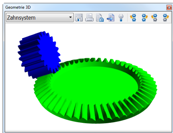
Bild 11. Schrägverzahntes Kronenrad im Parasolid-Viewer
