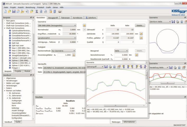
Bild 1. KISSsoft-Oberfläche
