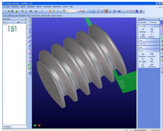
Bild 8. Zylinder Schnecke aus KISSsoft im Co-Create Modeling generiert
