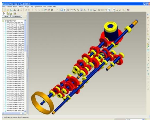
Bild 6. In Pro/ENGINEER importiertes Traktorgetriebe aus KISSsys
