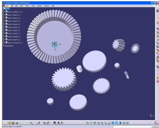
Bild 4. Zahnräder aus KISSsoft in CATIA generiert
