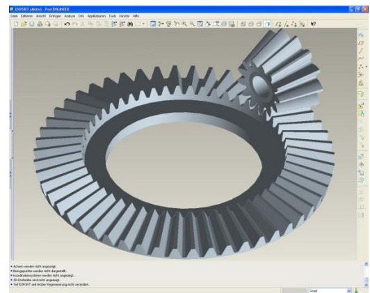
Bild 2. Kegelräder im Eingriff in Pro/ENGINEER
